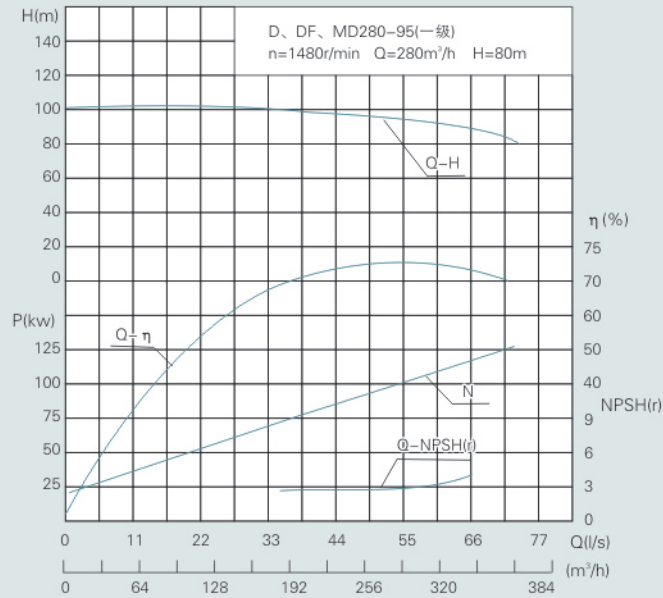
ZD、ZDG、ZDF、ZDY、ZMD 280-95型泵性能曲线和性能参数表 Performance Curve and Data Table for ZD, ZDG, ZDF, ZDY, ZMD 280-95
