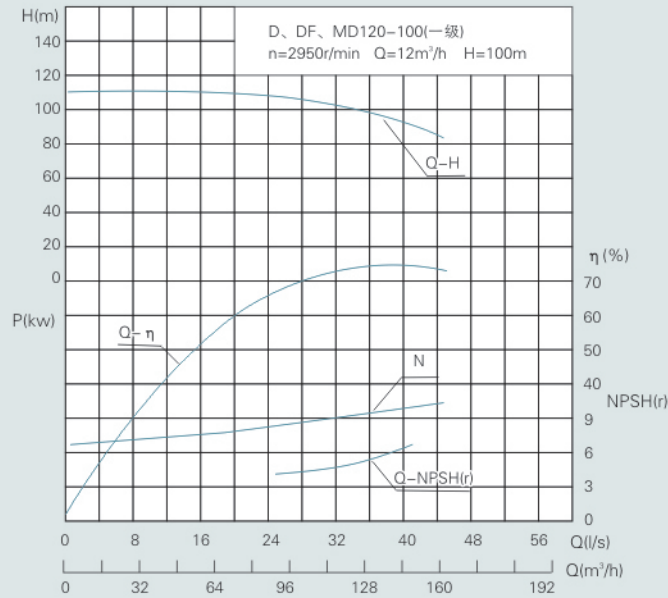
ZD、ZDG、ZDF、ZDY、ZMD 120-100型泵性能曲线和性能参数表 Performance Curve and Data Table for ZD, ZDG, ZDF, ZDY, ZMD 120-100
